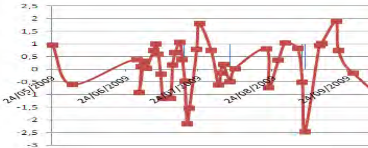
Figure 10 : Courbe des écarts de température de l'air
