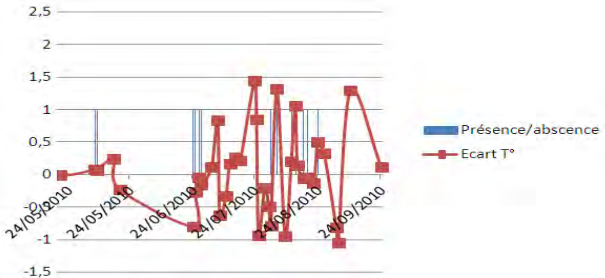
Figure 10 : Courbe des écarts de température de l'air
